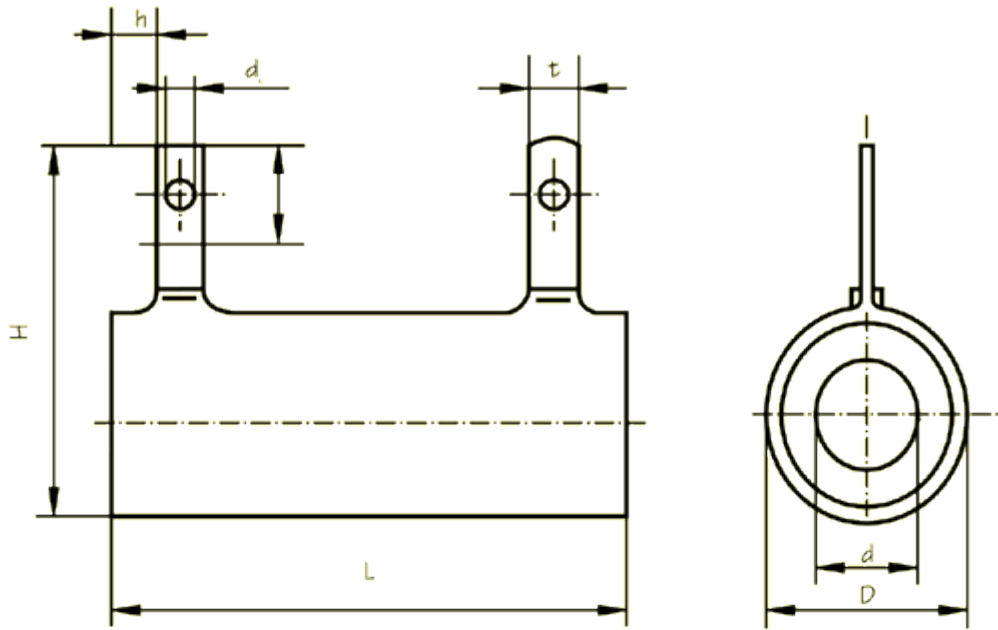
Rezystor DESW
